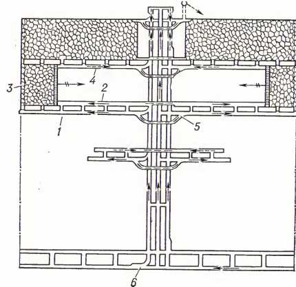
Рис. 11. Система разработки длинными столбами по простиранию: 1 — откаточный штрек; 2 — конвейерный ярусный штрек; 3 — разрезная печь; 4 — вентиляционный ярусный штрек; 5 — промежуточная приёмно-отправительная площадка; 6 — нижняя приёмно-отправительная площадка.
